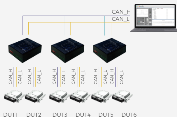
ETS6124-BR/CR级联图
