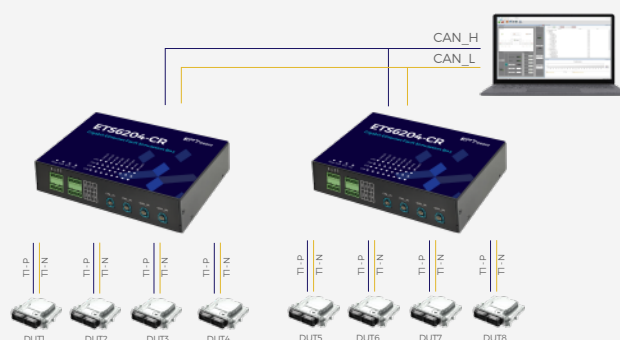
ETS6204-CR级联图
