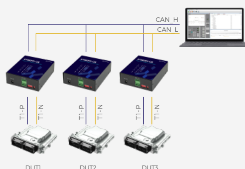
ETS6201-BR/CR级联图
